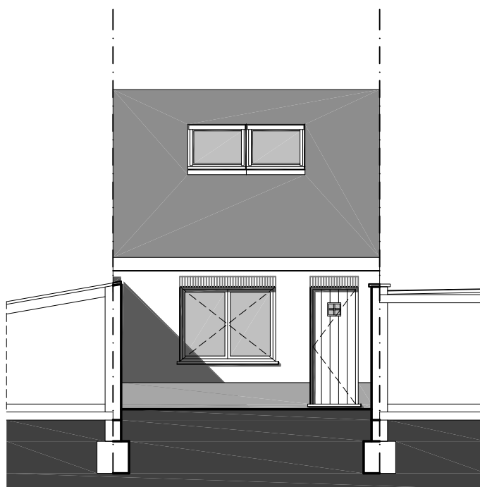
ACHTERGEVEL (garage)
