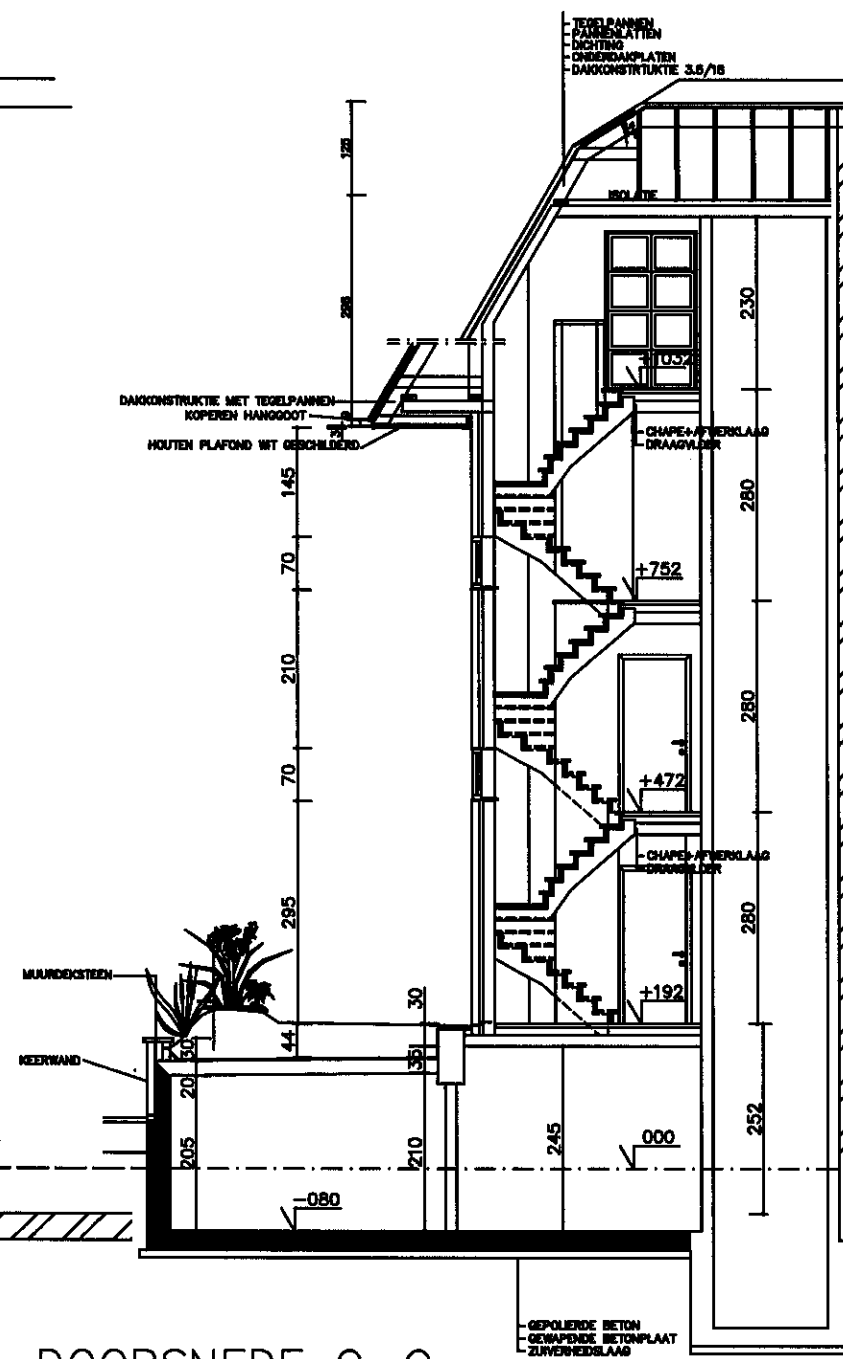
DOORSNEDE C-C
