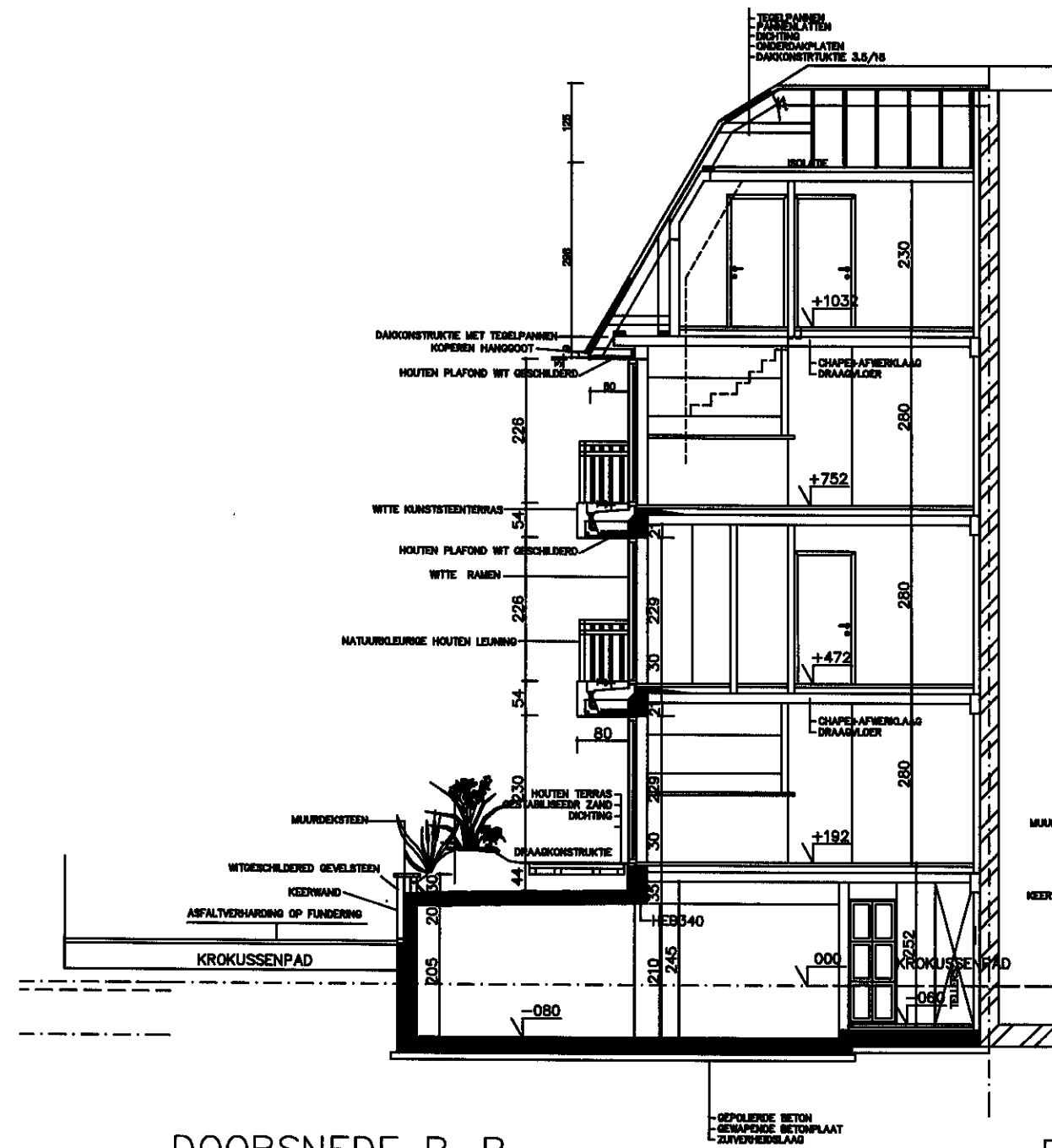
DOORSNEDE B-B
